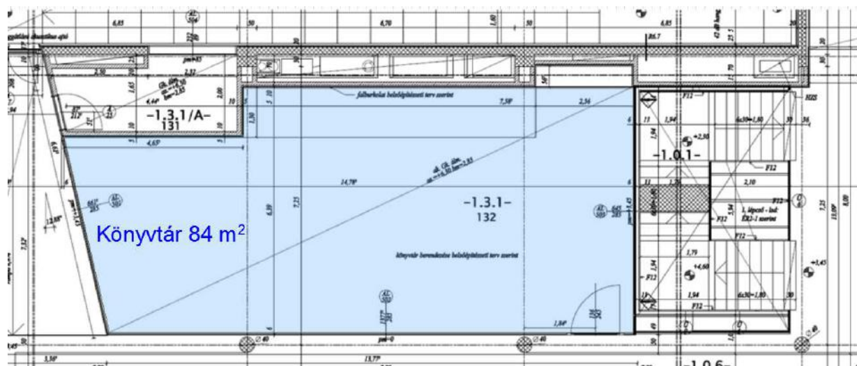
119. kép: Alaprajzi részlet, 1. emelet
