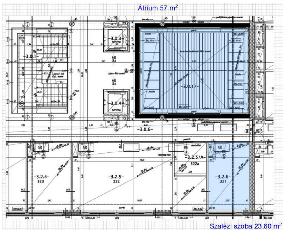
117. kép: Alaprajzi részlet, 3. emelet
