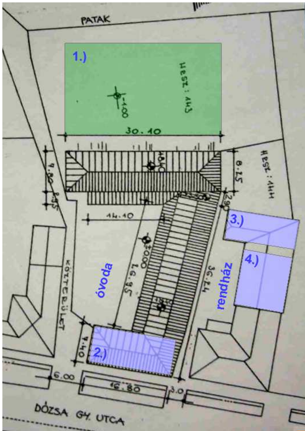
3.3.2 Helyszínrajz a létesítmények feltüntetésével
